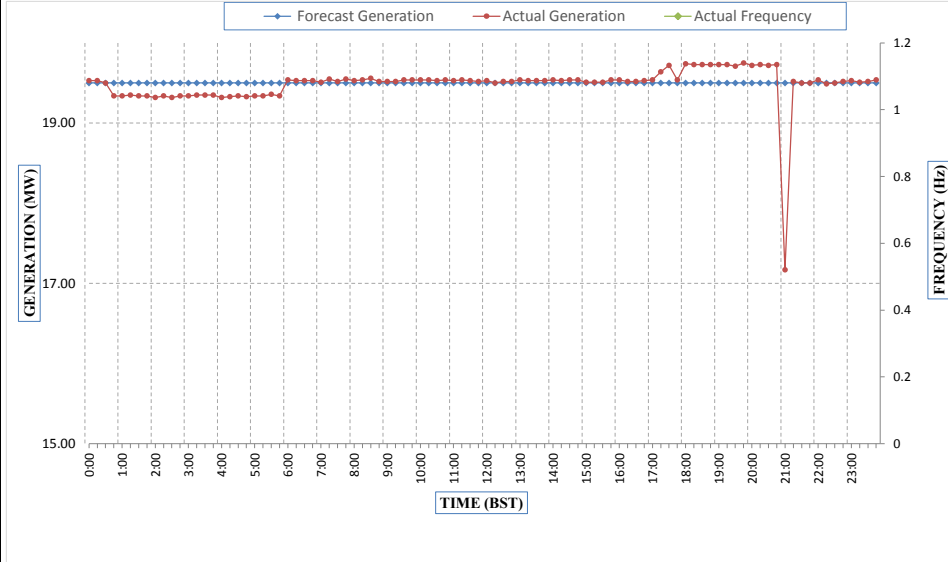
Forecast Generation & Actual Generation of Dagachhu(04-Feb-2018).
