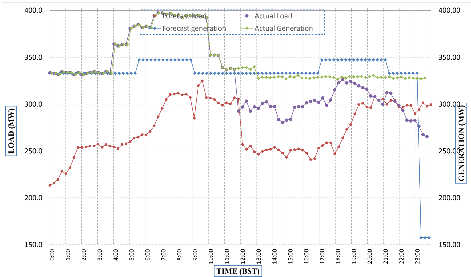
Forecast Generation & Load with Actual Generation & Load (15-Jan-2018).
