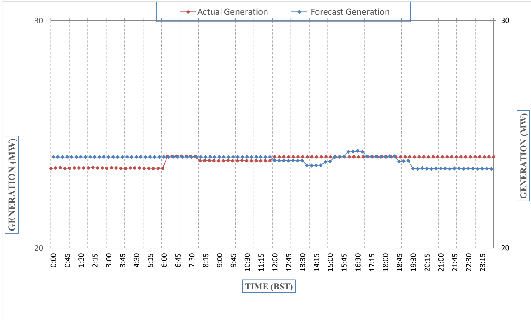
Scheduled Generation & Actual Generation of Dagachhu(03-Jan-2018).
