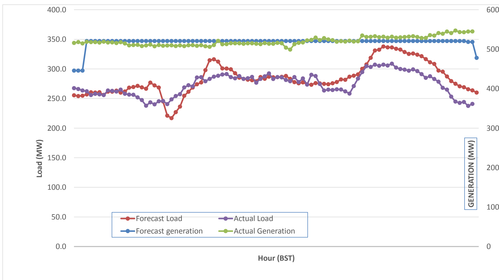
Forecast Generation & Load with Actual Generation & Load (27-Nov-2017).
